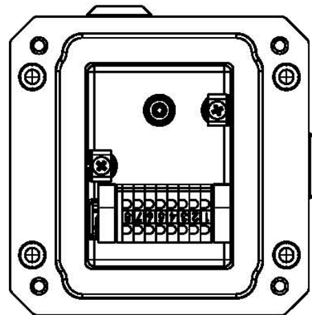
Fig. 4 DIN Rail in Base
